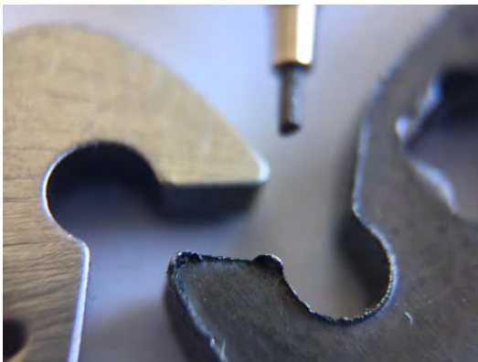
Bild Nr. 07-03 SY-WerkstückGrat.jpg Der partiell anfallende Massivgrat wird prozesssicher entfernt und die gesamte Teilekontur bei einem autonomen Durchsatz von über 14.000 Teilen pro Stunde gleichmäßig verrundet.
